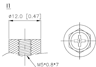
[M5 bolt & nut]
